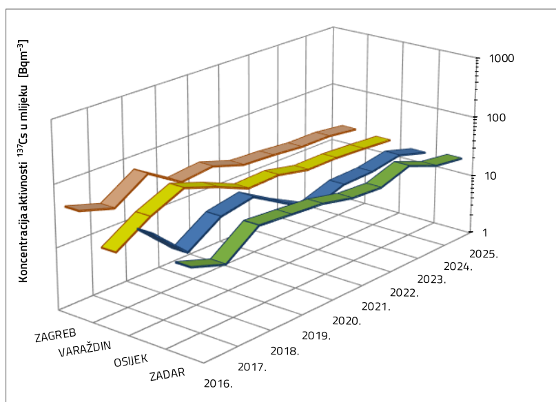
Slika 7. Srednje godišnje koncentracije aktivnosti 137 Cs u mlijeku zagrebačke, varaždinske, osječke i zadarske mljekare
