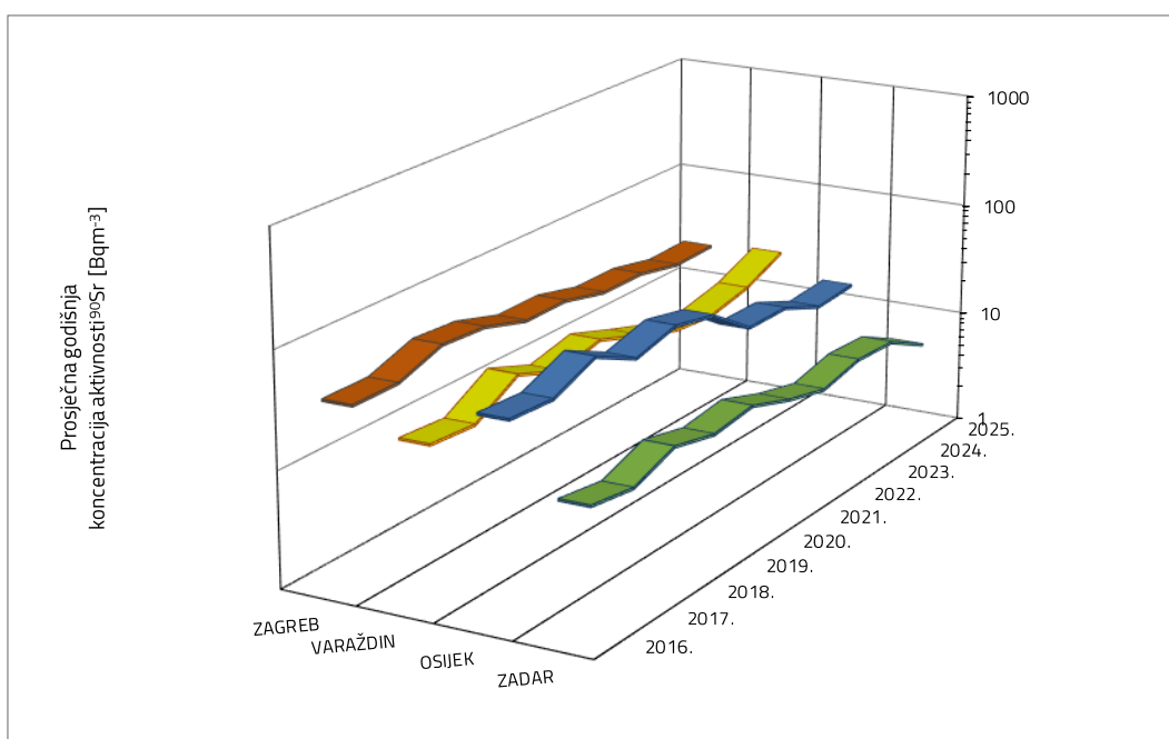
Slika 8. Srednje godišnje koncentracije aktivnosti 90 Sr u mlijeku zagrebačke, varaždinske, osječke i zadarske mljekare
