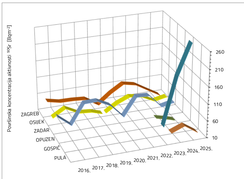
Slika 6. Koncentracije aktivnosti ^{90}\text{Sr} [ \text{Bq}/\text{m}^2 ] izmjerene u prvim slojevima neobrađenog tla
